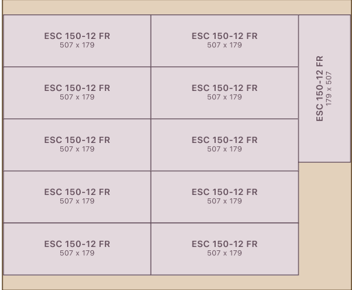
Pallet 1200 x 1000 mm, top view, 11 cartons per layer
